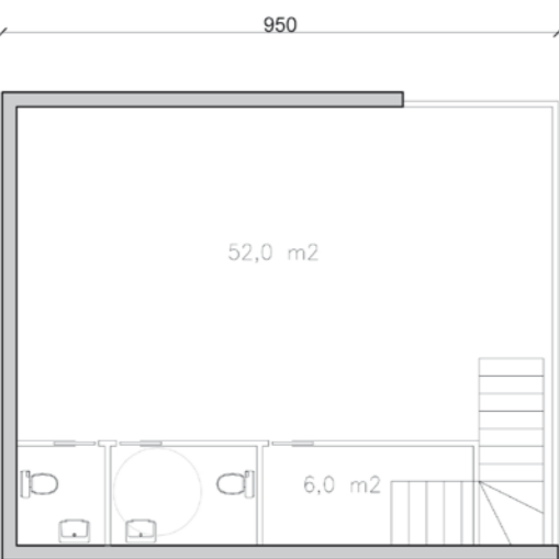
TLOCRT PRIZEMLJA
