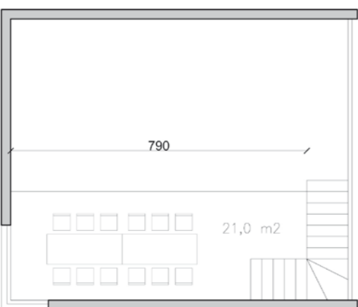
TLOCRT GALERIJE
