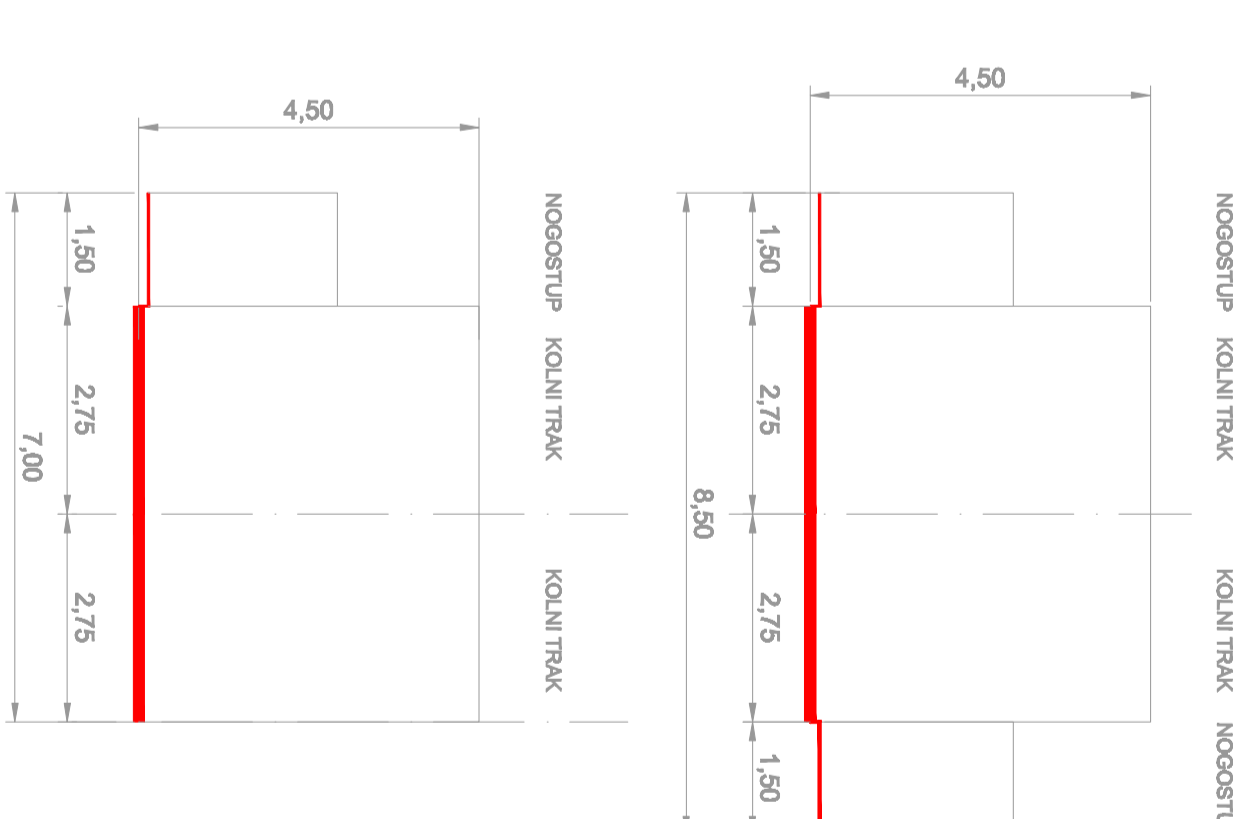
PLANIRANI POPREČNI PRESJECI PROMETNICA MABELO 1:100
