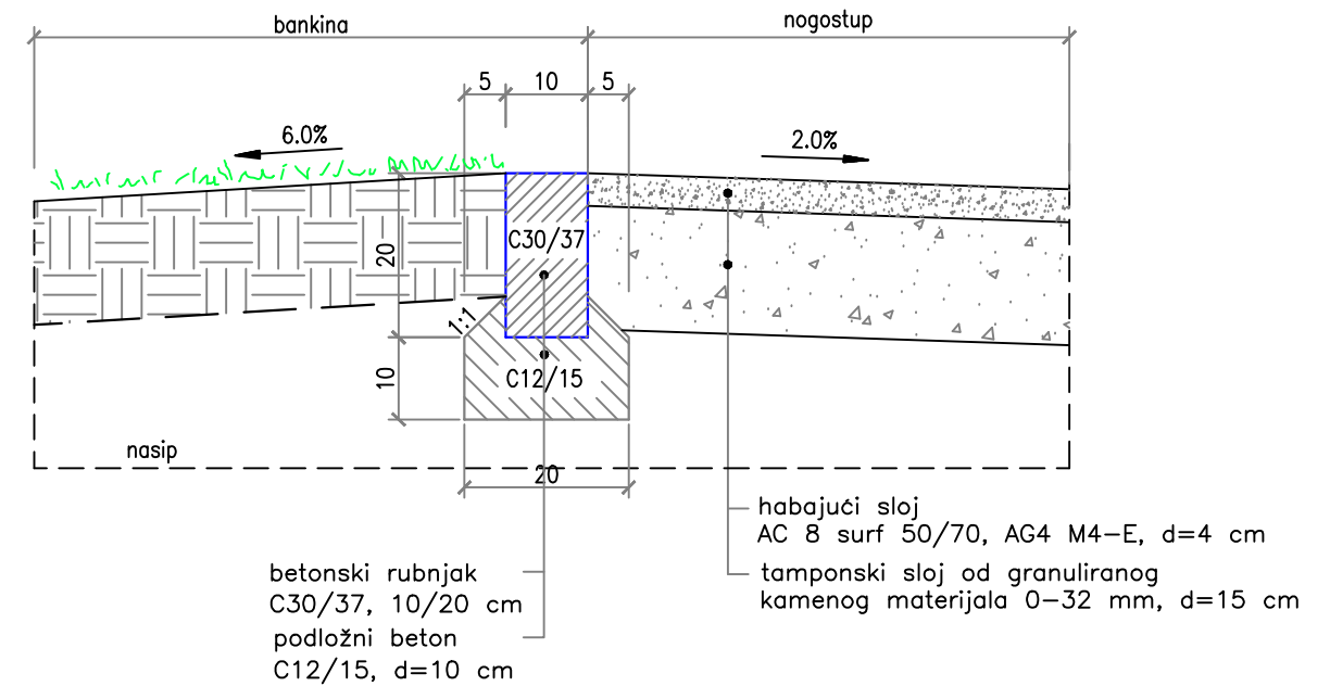
DETALJ RUBNJAKA 10/20 cm
