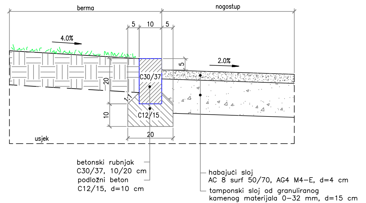
DETALJ BETONSKOG RUBNJAKA
