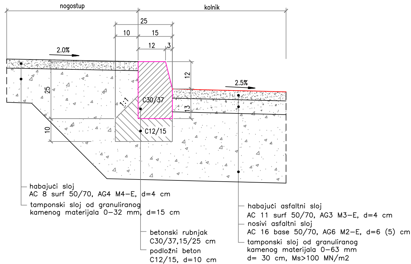
DETALJ RUBNJAKA 15/25 cm
