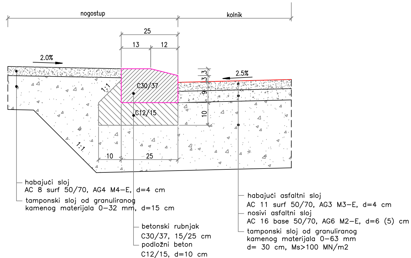
DETALJ POLOŽENOG RUBNJAKA
